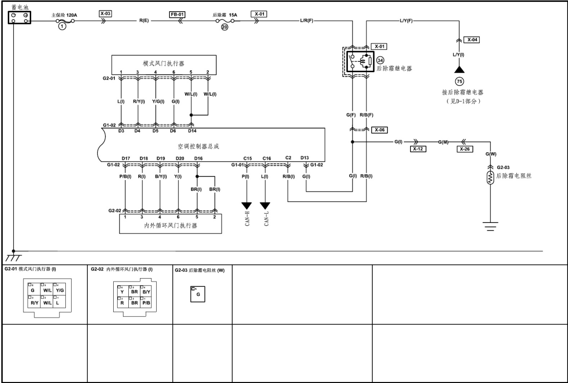
加热和空调系统(后除霜)
