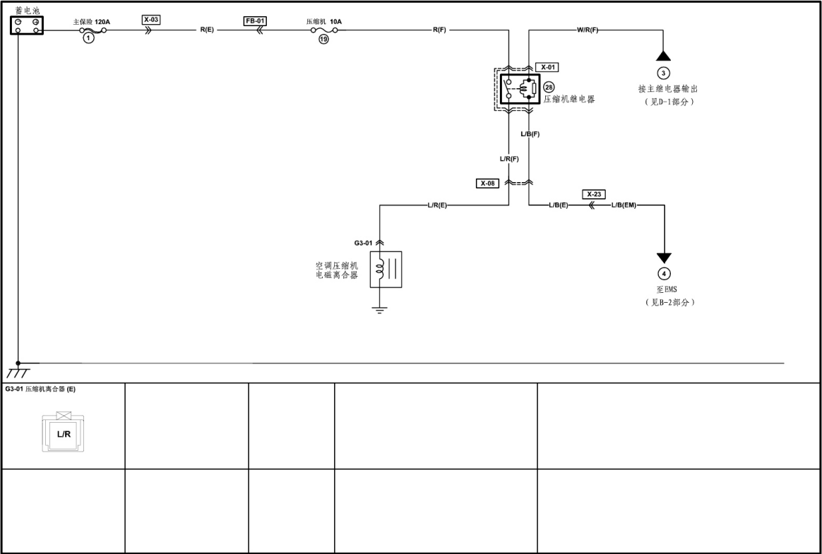
加热和空调系统(空调压缩机)
